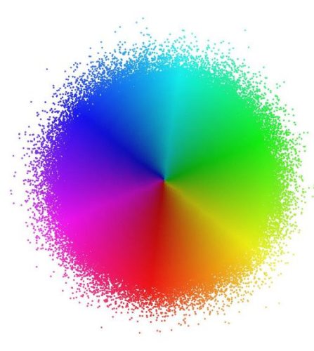
LeJEPa f(x)
