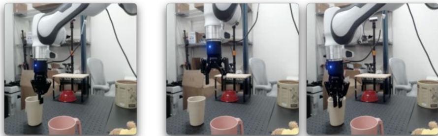
VJEPA 2.1
